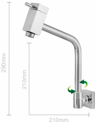
4911 - C22 Torneira Piazza Giratória Parede Tubo Redondo 3/4" 1/4 de Volta M18
