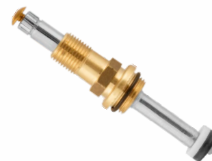
17180 - PISTÃO AMARELO 17181 - PISTÃO CROMADO Reparo Vedante M18 p/ Registro de Pressão Rosca 2
