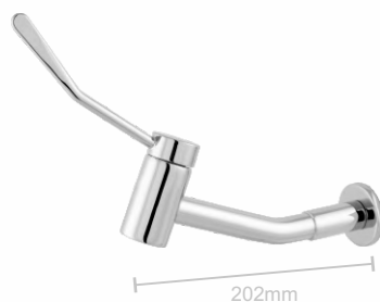
2296 Torneira Lavatório Clínica Parede com Arejador Fixo 1/4 de Volta M22 - Tubo 13/16"
