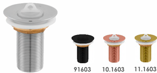
1603 - Latão Válvula para Lavatório ou Pia 70mm 7/8"
