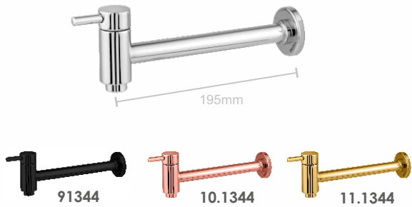
1344 - Arejador Fixo 1345 - Arejador Articulado Torneira Lavatório ou Cozinha Vernazza Parede 1/4 de Volta M18 Tubo 3/4" - Acabamentos: C28, C70
