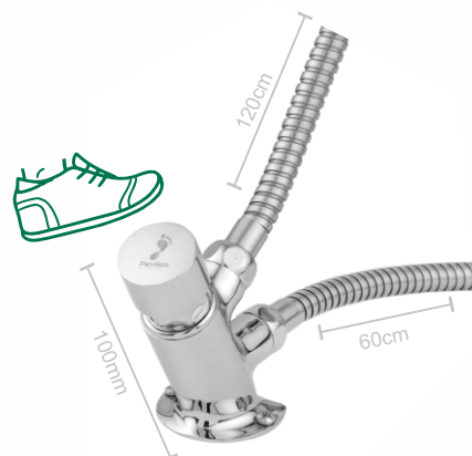
11800 Pedal Acionador com Fechamento Automático
