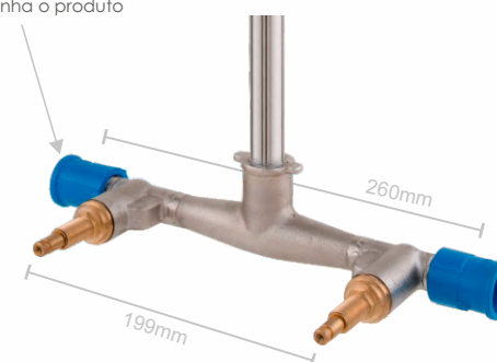
2920 - 1/4 de Volta 2922 - Vedante Base para Misturador Registro de Pressão 1/2" - M25
