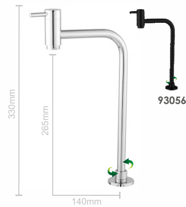
3056 - Arejador Fixo Torneira em Inox Giratória Bancada 1/4 de Volta M18 Cano 5/8" Acabamento Único
