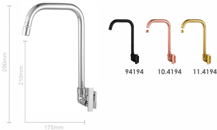
4194 - C73 Torneira Cozinha Parede Giratória Cano 3/4" com Arejador Articulado 1/4 de Volta M18
