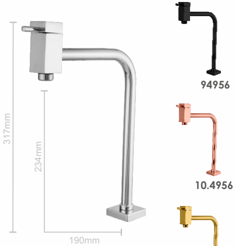
4956 - C22 Torneira Piazza Fixa Bancada Tubo Redondo 3/4" 1/4 de Volta M18
