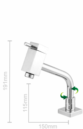
4920 - C22 Torneira Piazza Giratória Bancada Tubo Redondo 3/4" 1/4 de Volta M18
